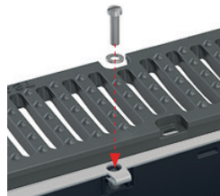
קביוע באמצעות ברגים
